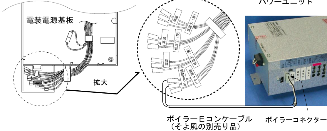
ボイラーEコン接続例(ノーリツGH712Wの場合)
